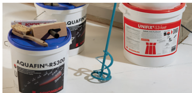
Системные компоненты для гидроизоляции в сочетании с плиткой (на изображении AQUAFIN-RS300 и UNIFIX-S3-Fast).
